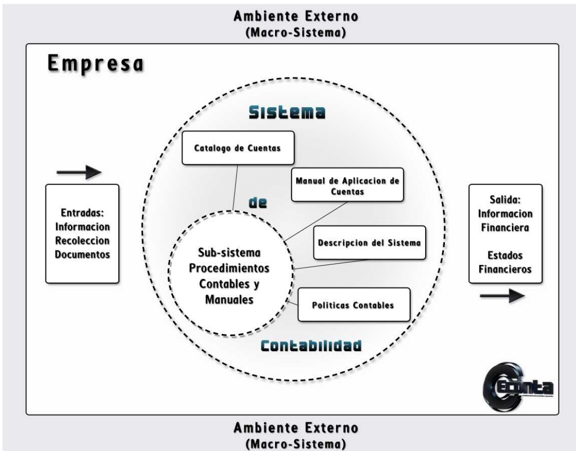
Figura 4. Sistema Contable.
